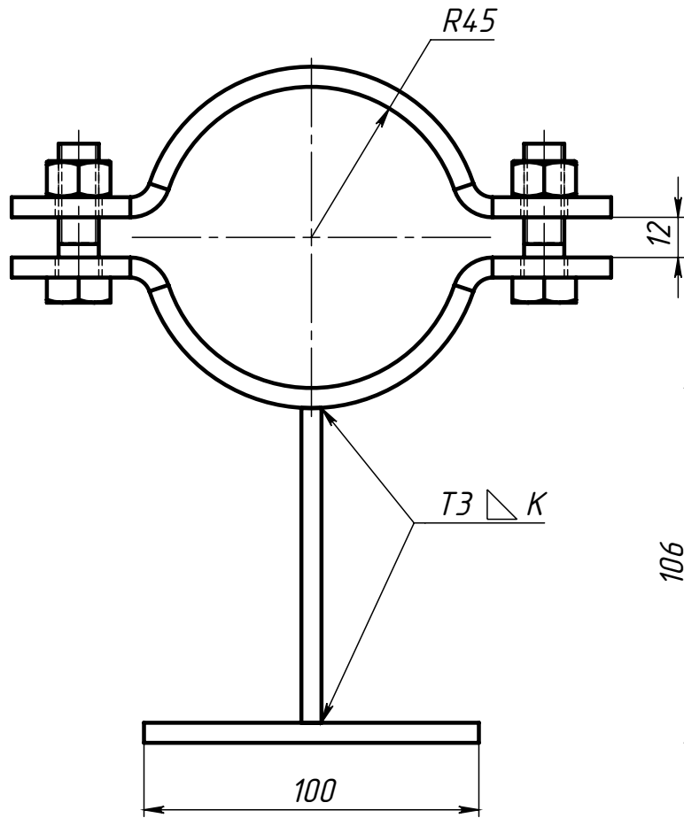
Поз.3 (Полухомут)
