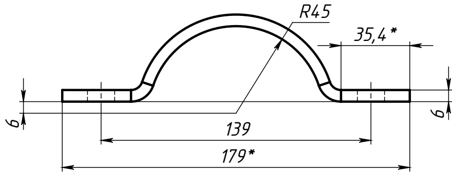
Поз.3 (Полухомут) развертка
